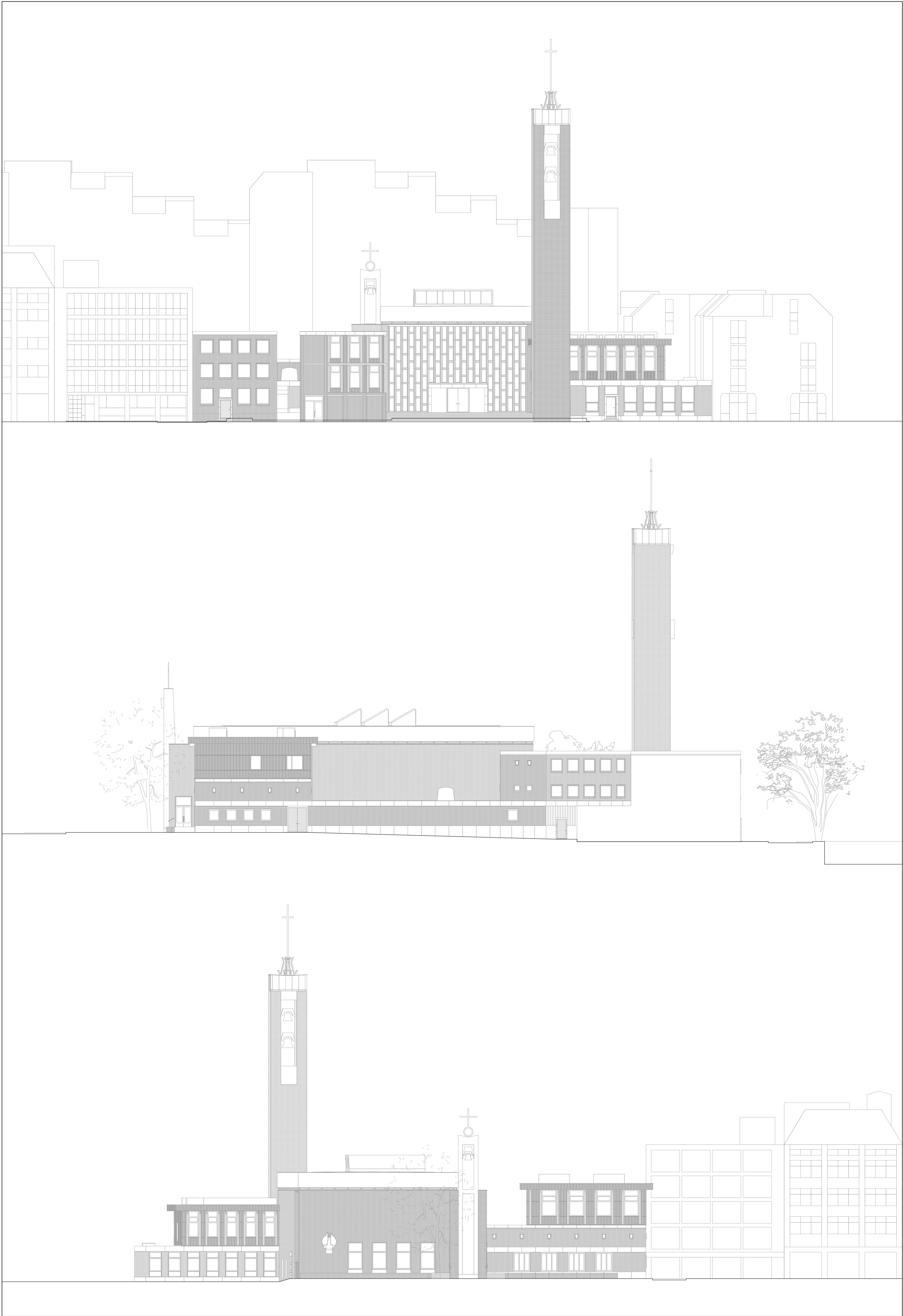
Art Complex Het Steiger elevations - new situation 1:200
