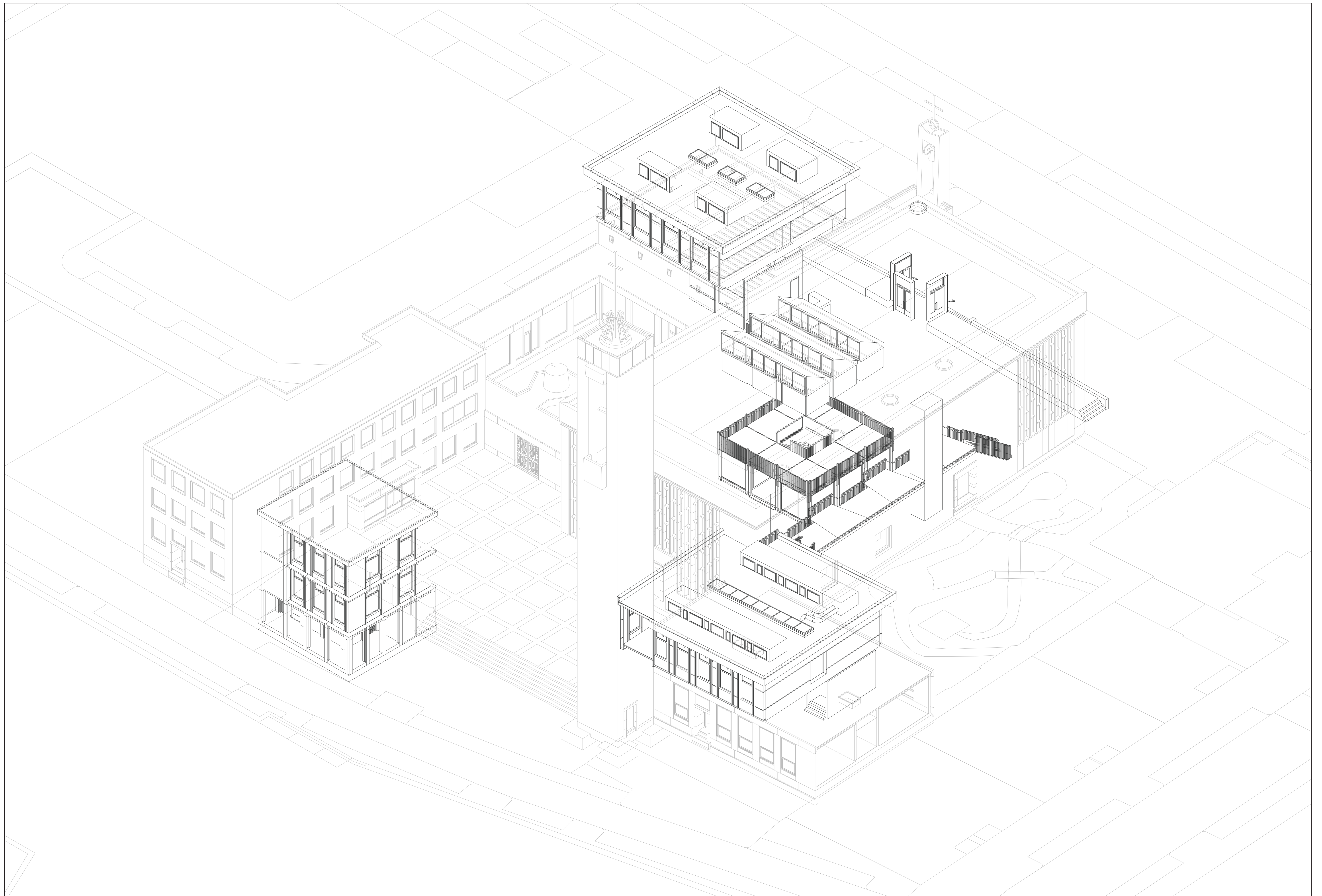
Art Complex Het Steiger overview of all design interventions 1:200
