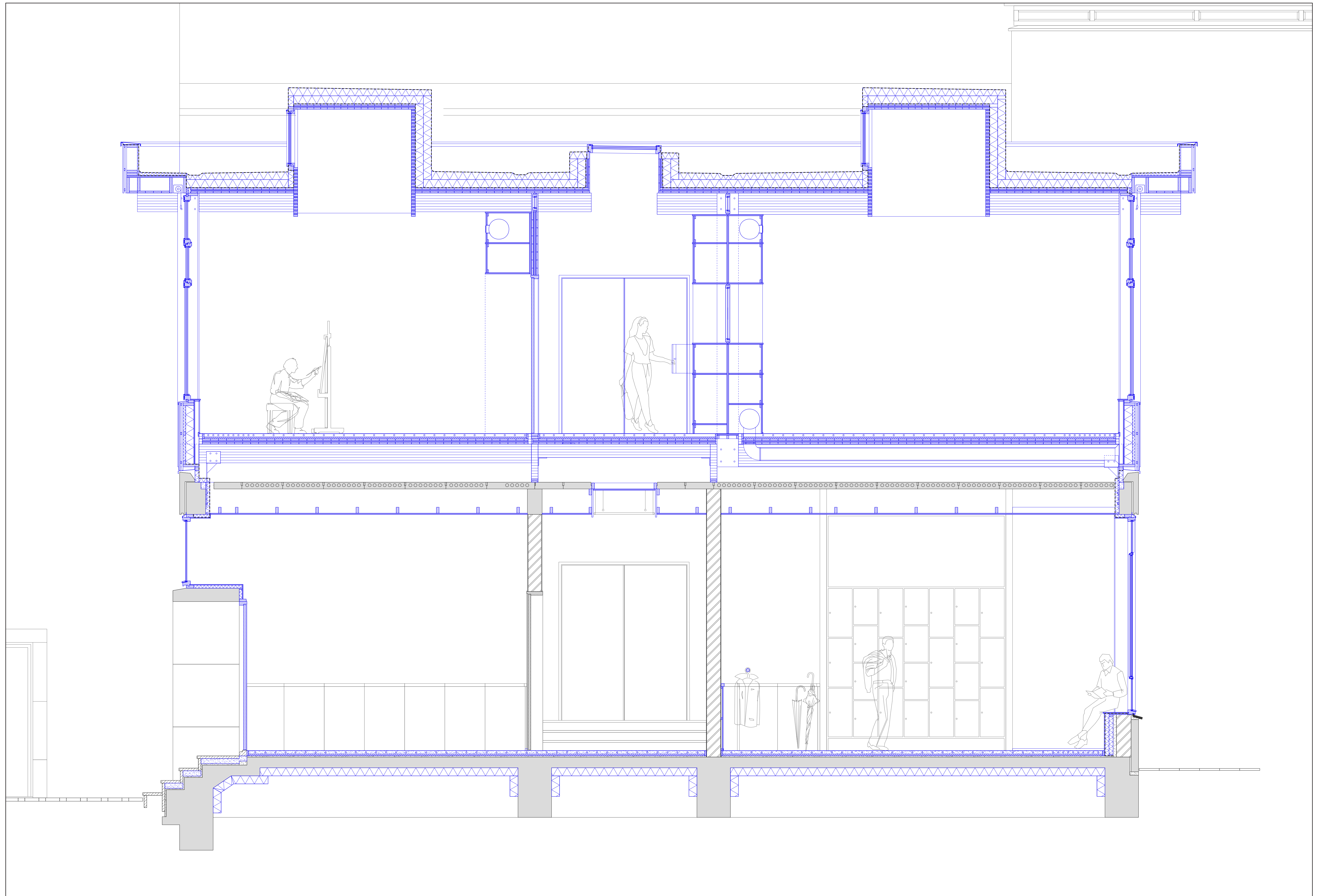
Art Complex Het Steiger fragment section 1:25
