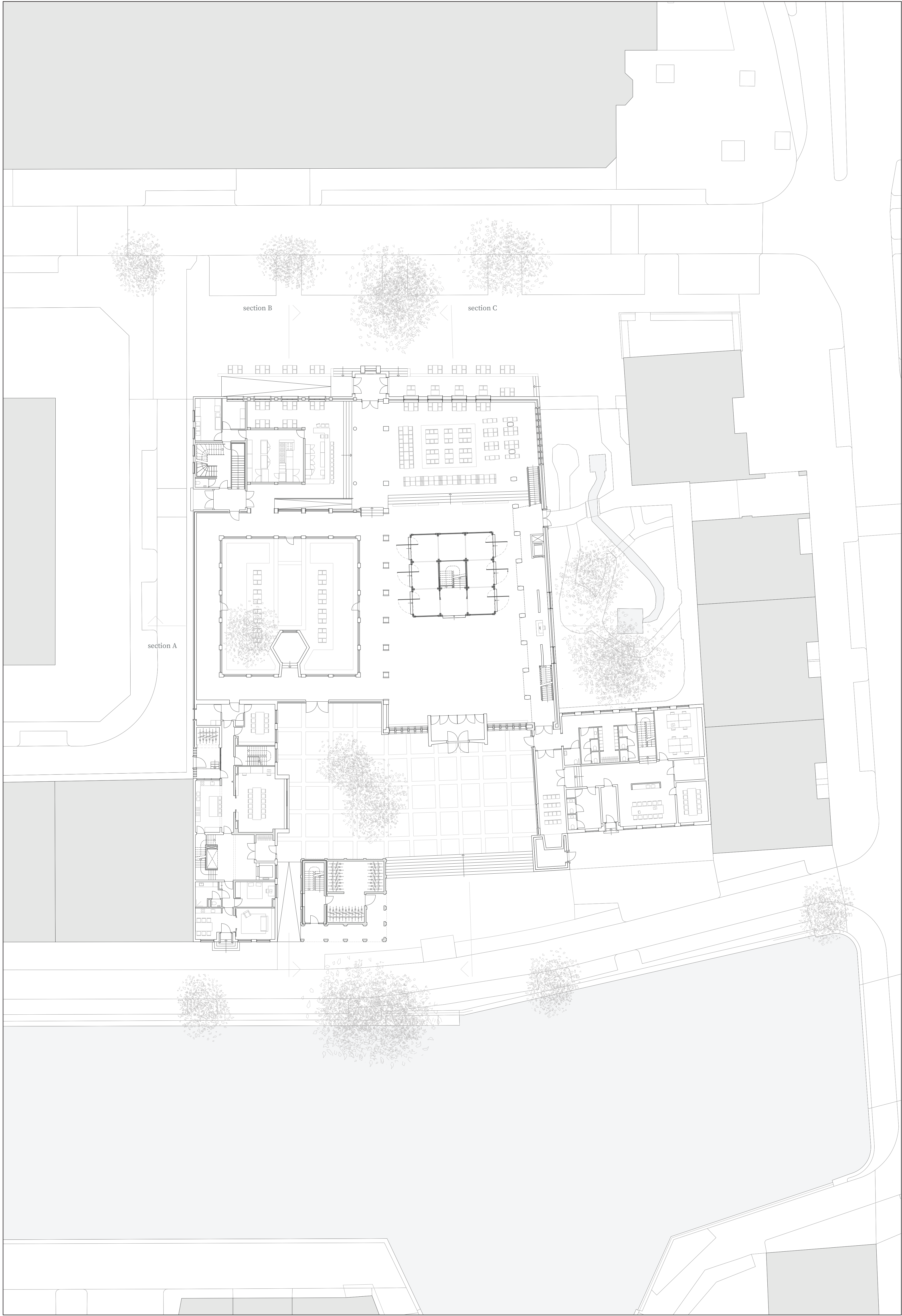
Art Complex Het Steiger floor plan level 00 - new situation 1:200
