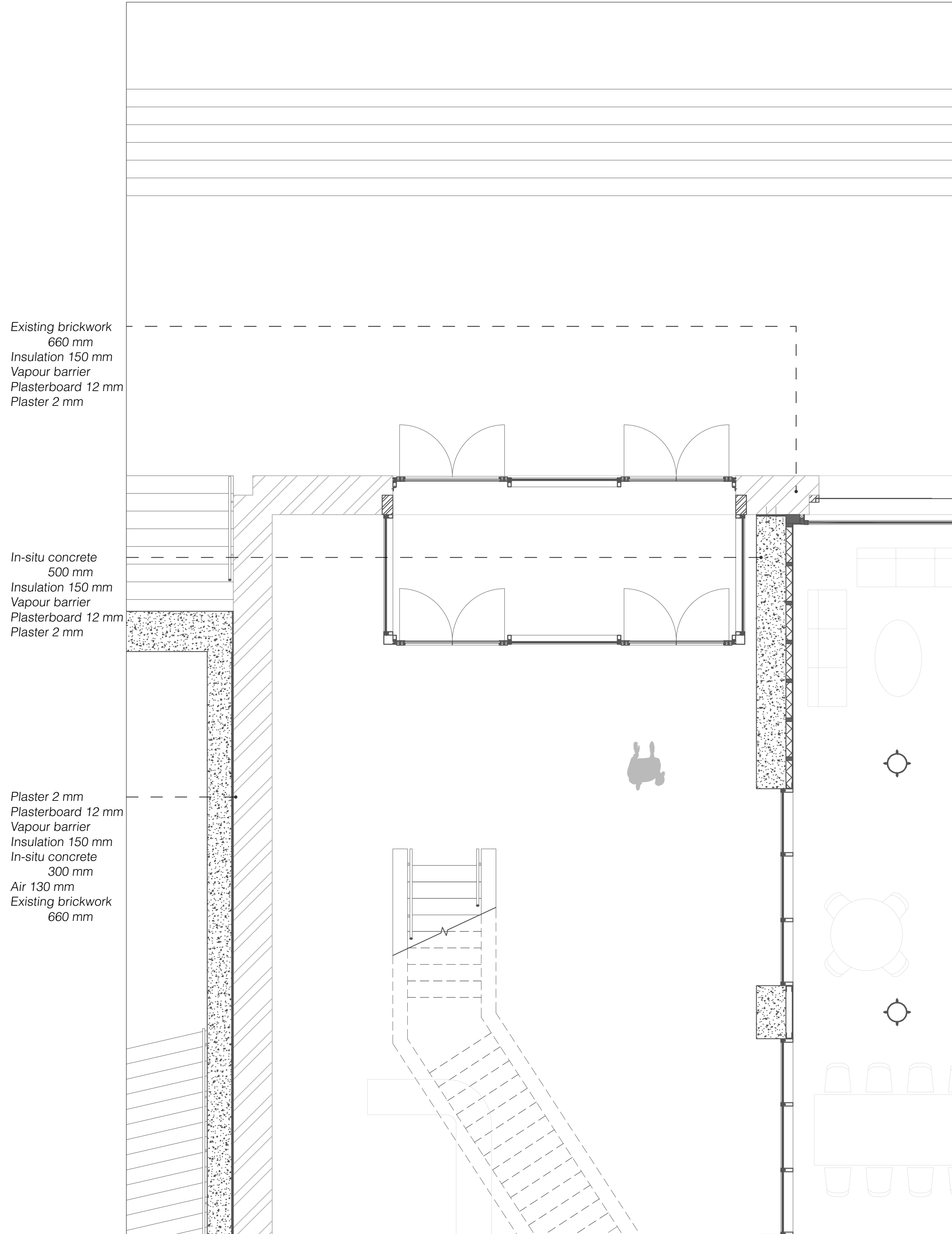
1:50 Plan
