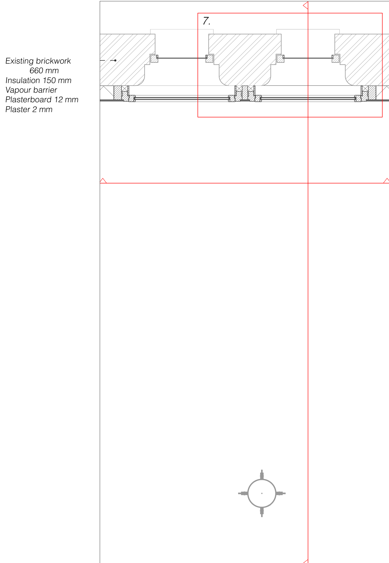
1:20 Plan
