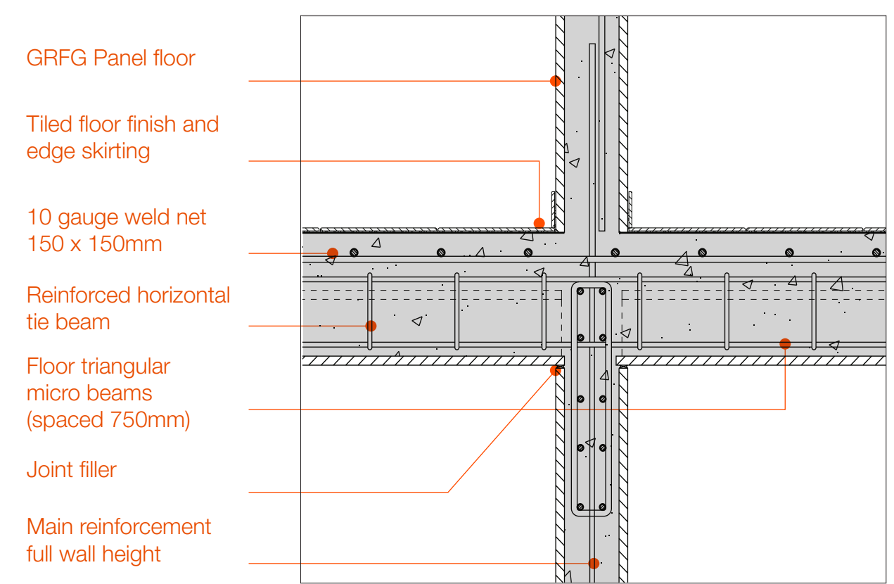
STRUCTURAL D10.
