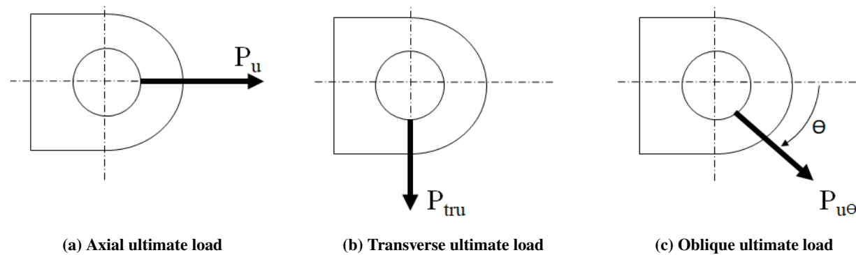
Fig. 7 Lug loading.
