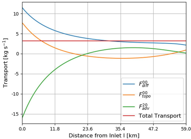
(a) E1–Transport Contributions
