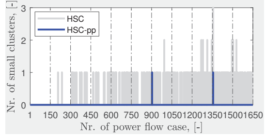
(d) case2869pegase test network
