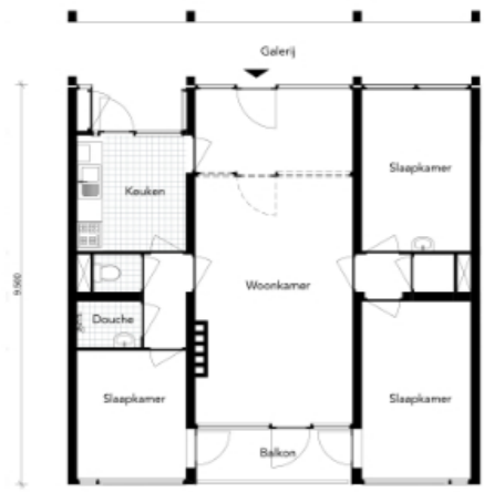
WONING PLATTEGROND - BESTAAND
