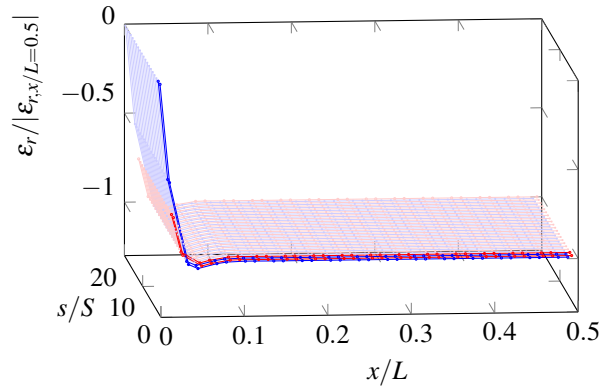
(d) (20,0) zigzag
