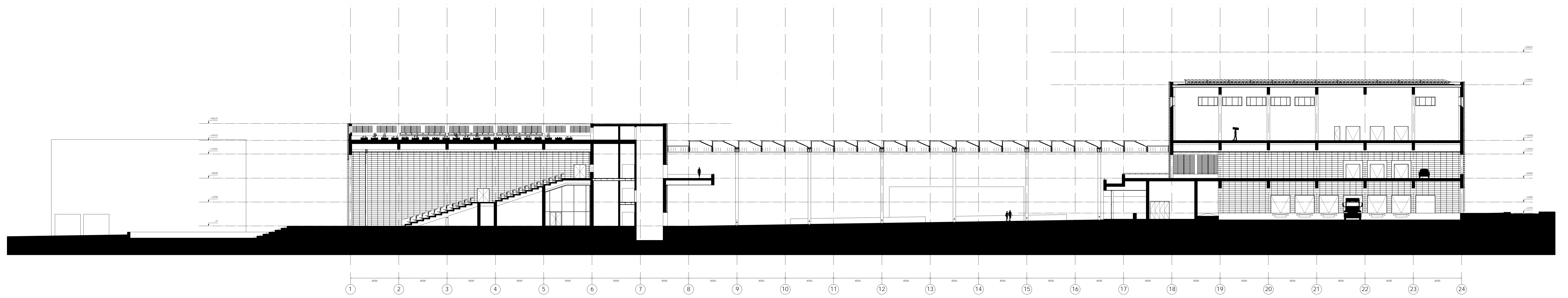
LONGITUDINAL SECTION 1 1:250
