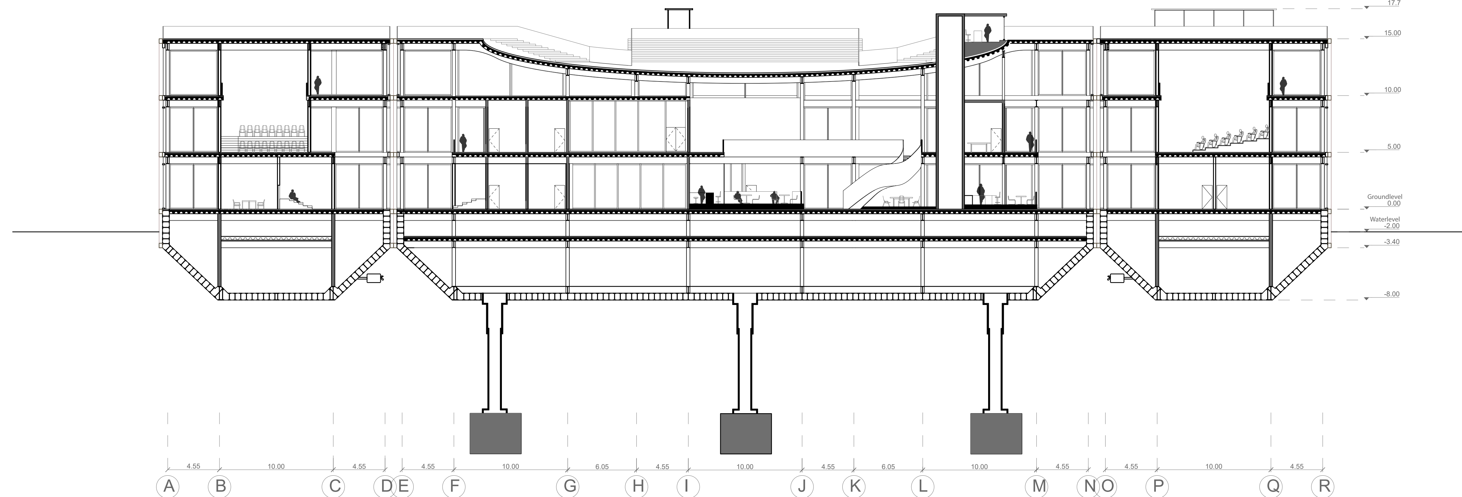
B-B Section - Cinema - 1:200
