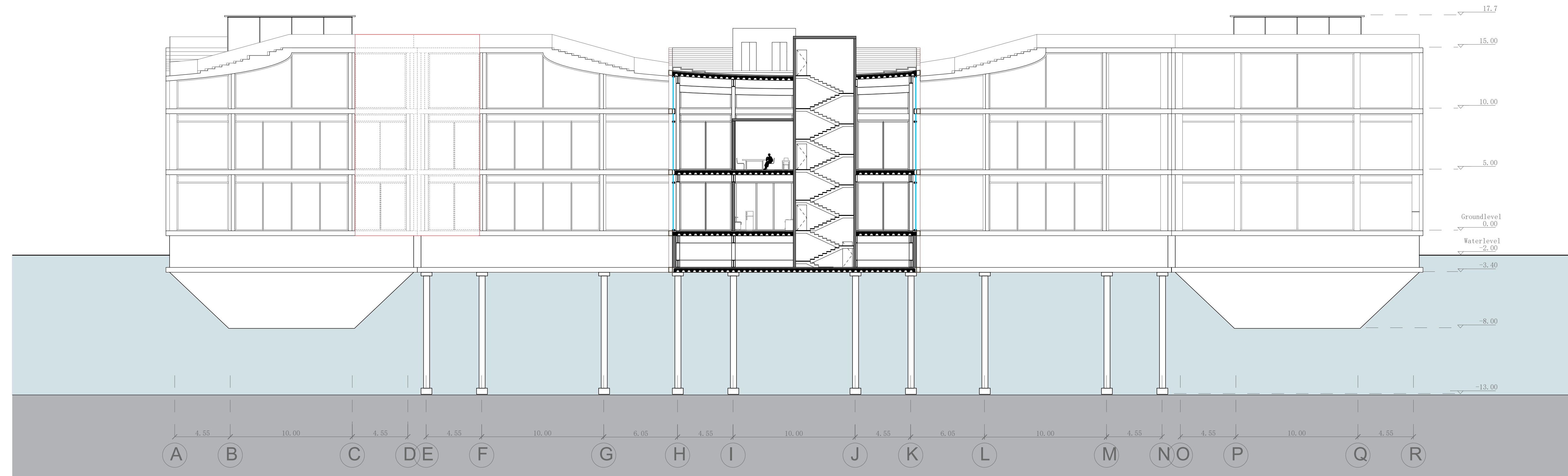
A-A Section - Cinema - 1:200
