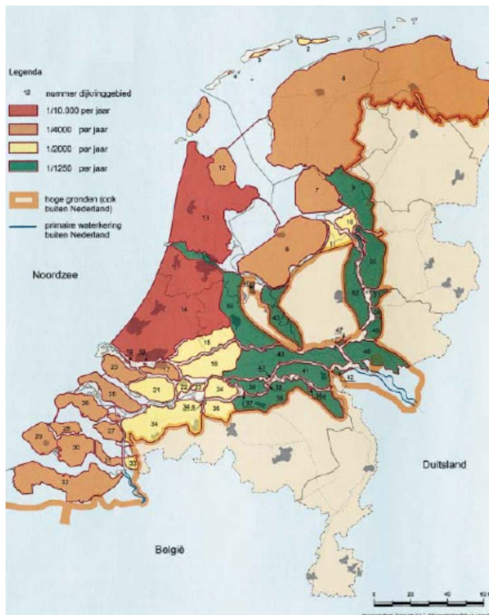
Kaart 6: Nederlandse dijkringgebieden en veiligheidsnormen, exclusief de dijkringgebieden en kades langs de Maas ten zuiden van Nijmegen (Waterwet, Bijlage I)
