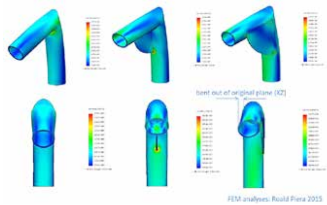
Afbeelding 7 Secundaire buiging als gevolg van een asymmetrisch versterkt knooppunt. (Roald Piers)
