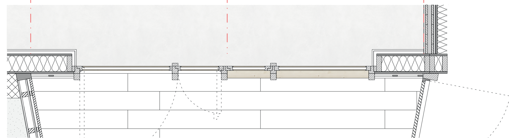
Horizontal fragment back side | 1 : 20
