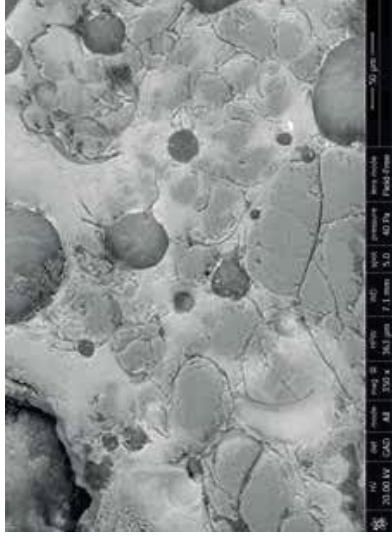
Abbeelding 6b: Teugetteerd elektronen beeld van een slijplaat, waarin het glas (lichtgrijs) zichtbaar is tussen de siltkorrels (donkergrijs).
