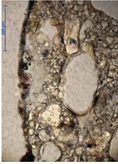
Abbeelding 6a: Microscopische foto van een slijplaat van de buitenkant van één van de kroesjes (nr. 11). Alleen siltkorrels en gesmolten materiaal (glas) zijn zichtbaar. De rode vlek middenboven is waarschijnlijk het gevolg van het oplossen van kleine hoeveelheden koper in het glas.
