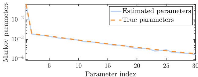
Fig. 4. Markov parameter estimation
