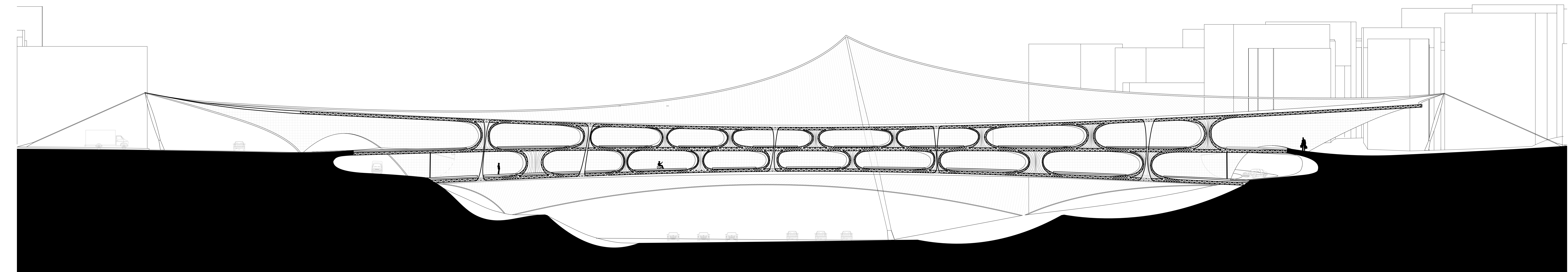
Longitudinal Section 1:200
