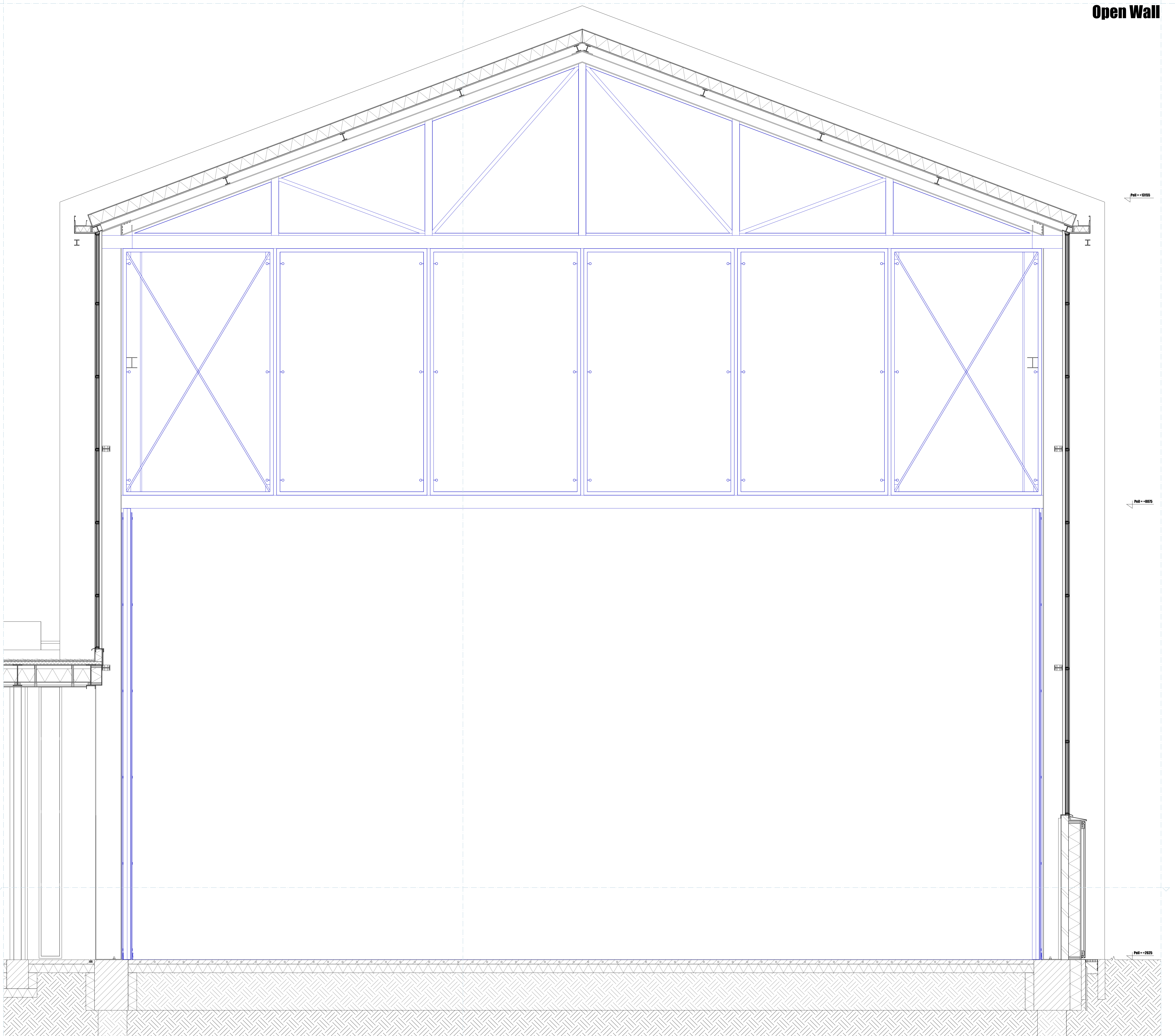
Longitudinal Vertical Section 1:20
