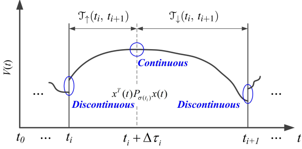
Fig. 1. The Lyapunov function (5).
