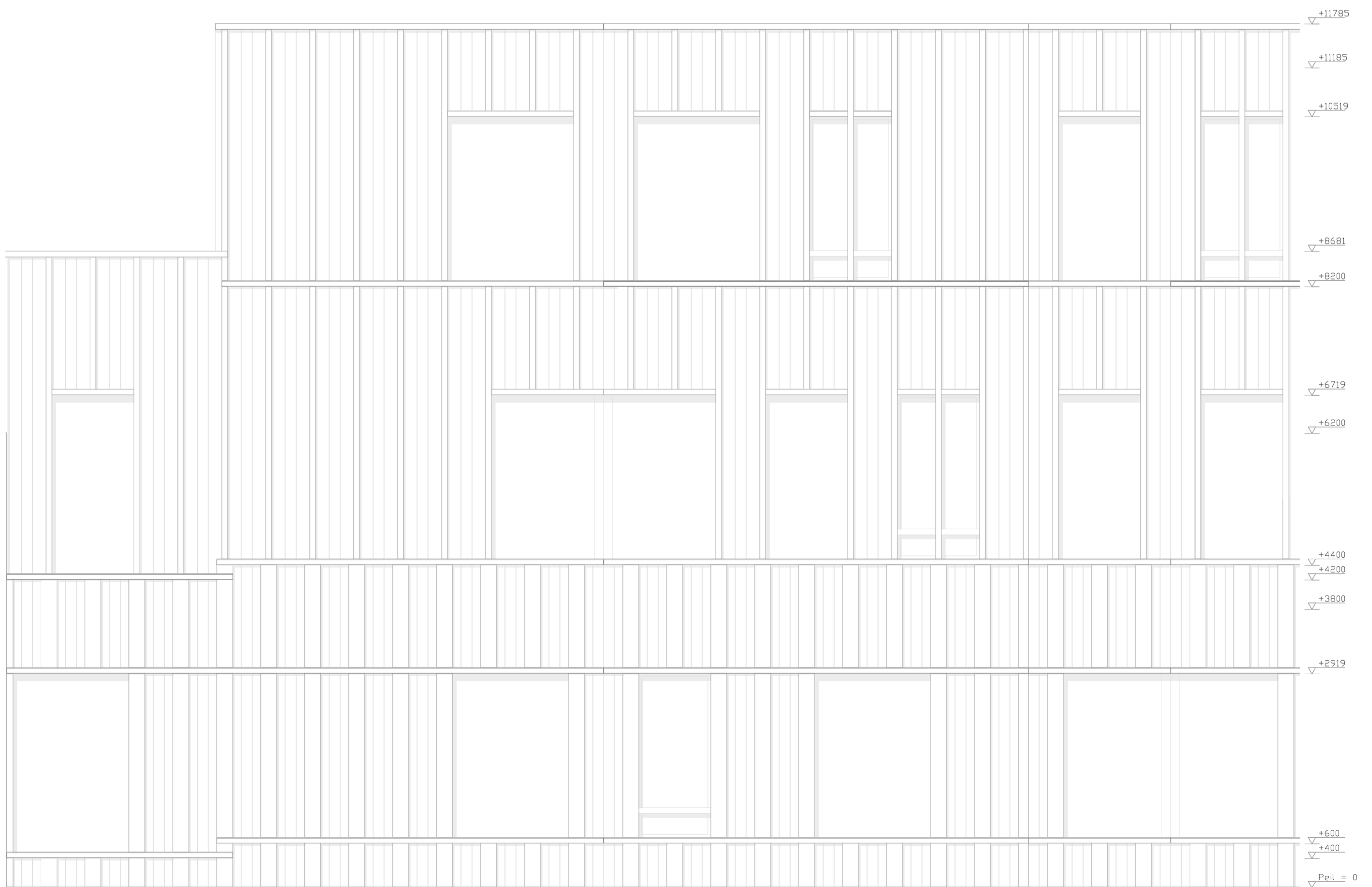
Gevelaanzicht
