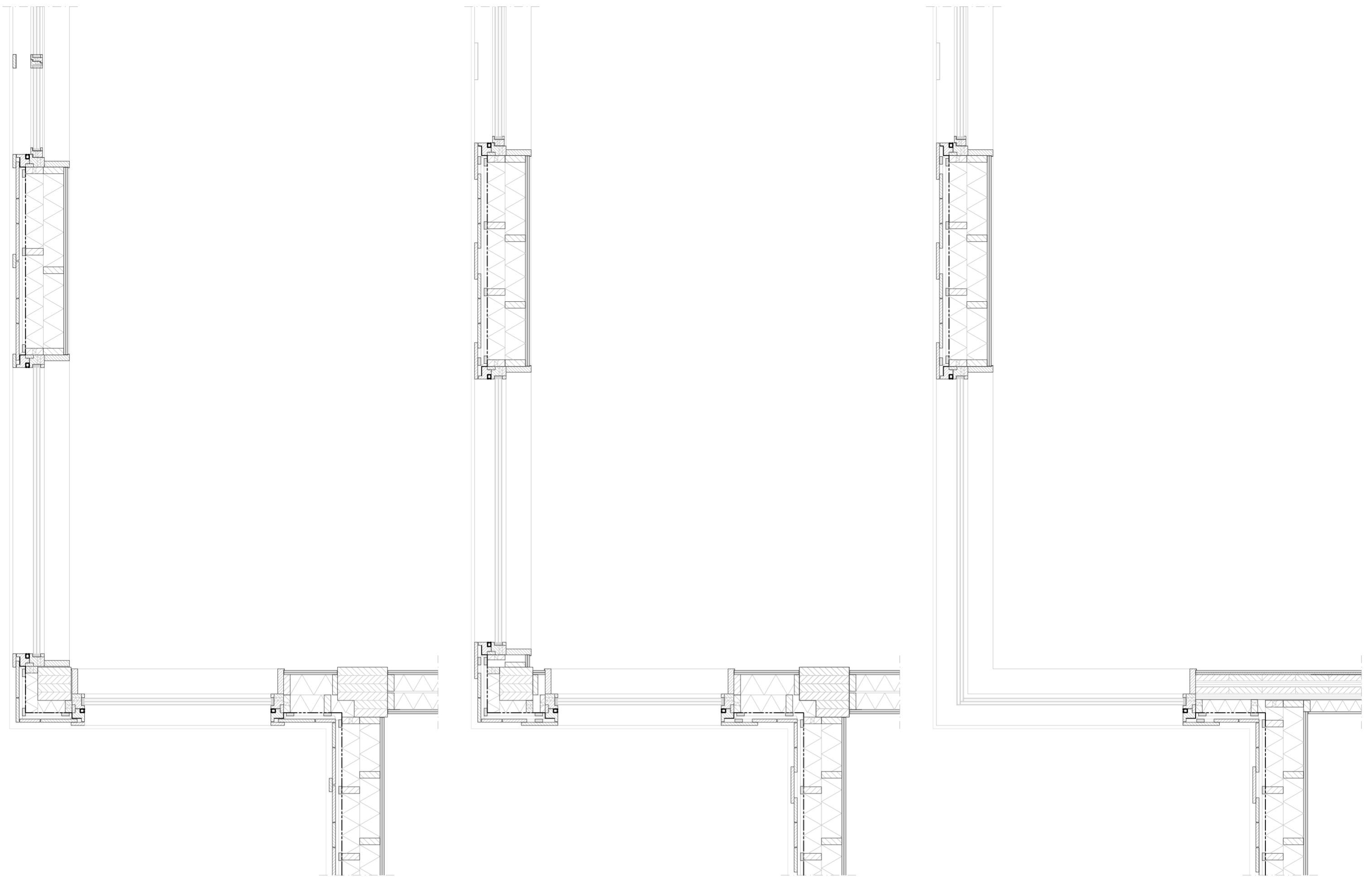
Geveldoorsnede horizontaal
