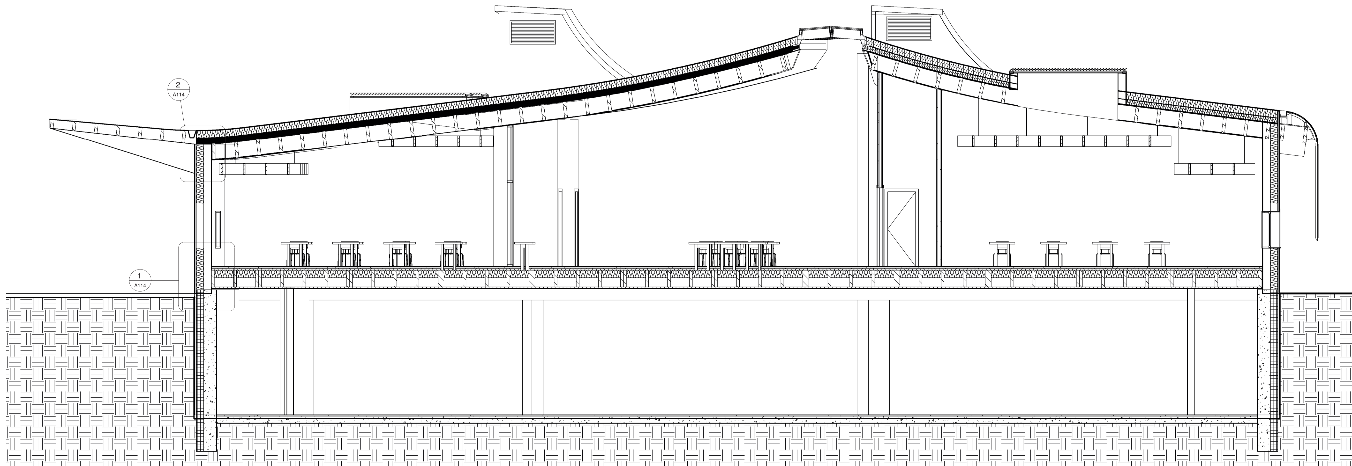
2 Section 5 50 1 : 50
