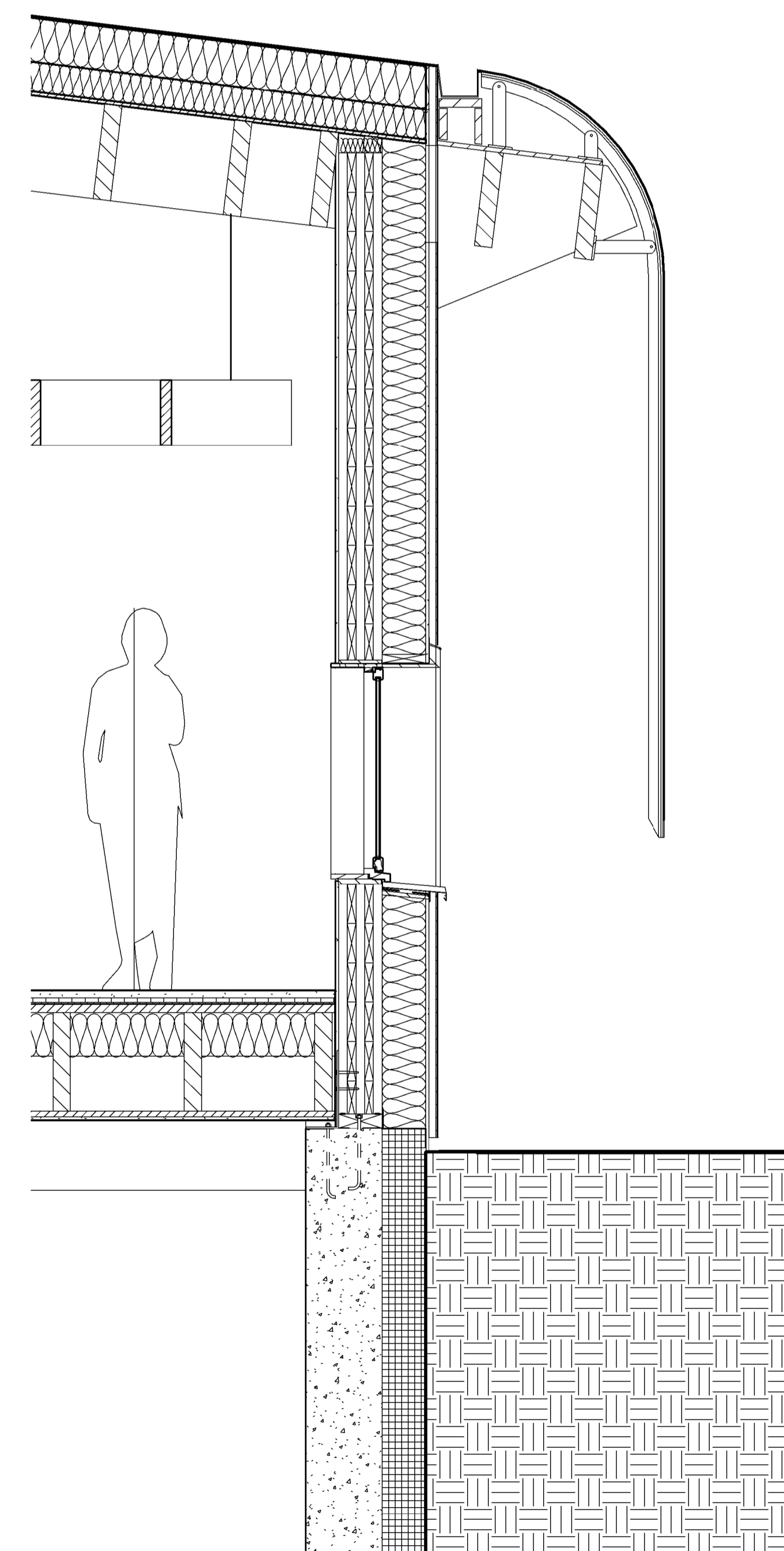
1 Section 5 50 20 1 : 20
