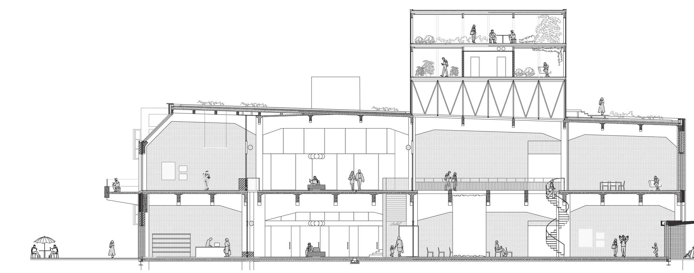
doorsnede bb | schaal 1:200
