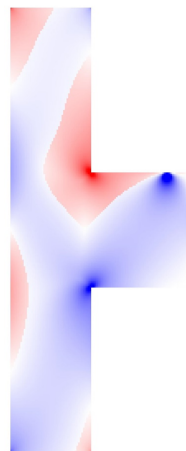
(b) Case II: Corbel (mesh size: 10 mm)
