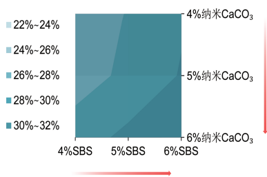
图 15 不同百分比的纳米 \text{CaCO}_3 /SBS 复合抑制剂的减排效果 [25]
