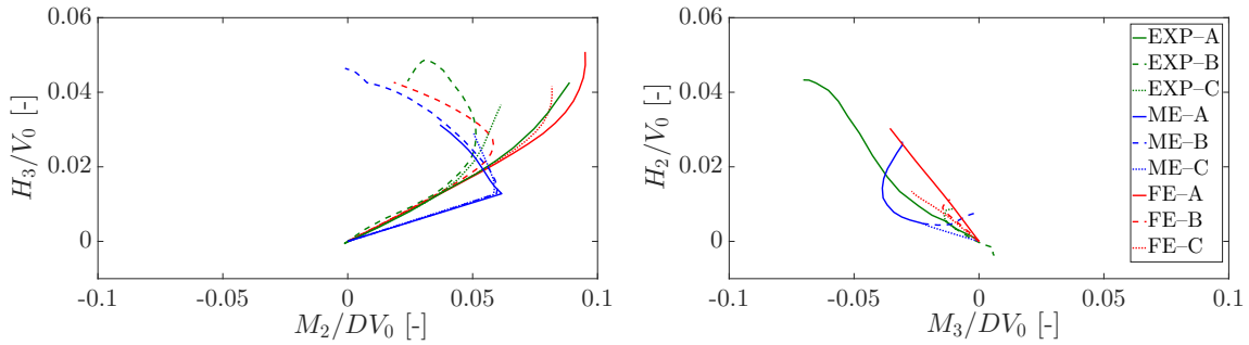
(a) horizontal-moment 1 ( H_3/V_0 - M_2/DV_0 ) (b) horizontal-moment 2 ( H_2/V_0 - M_3/DV_0 )
