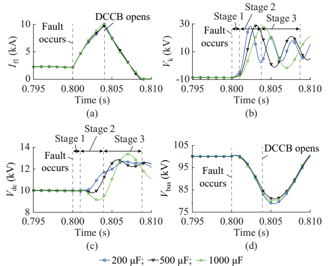
Fig. 18. Simulation results with different C_r . (a) I_{f1} . (b) V_k . (c) V_{dc} . (d) V_{bus} .
