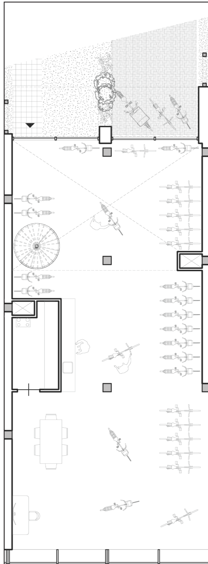
NouJIJ! - bike shop 1:100
