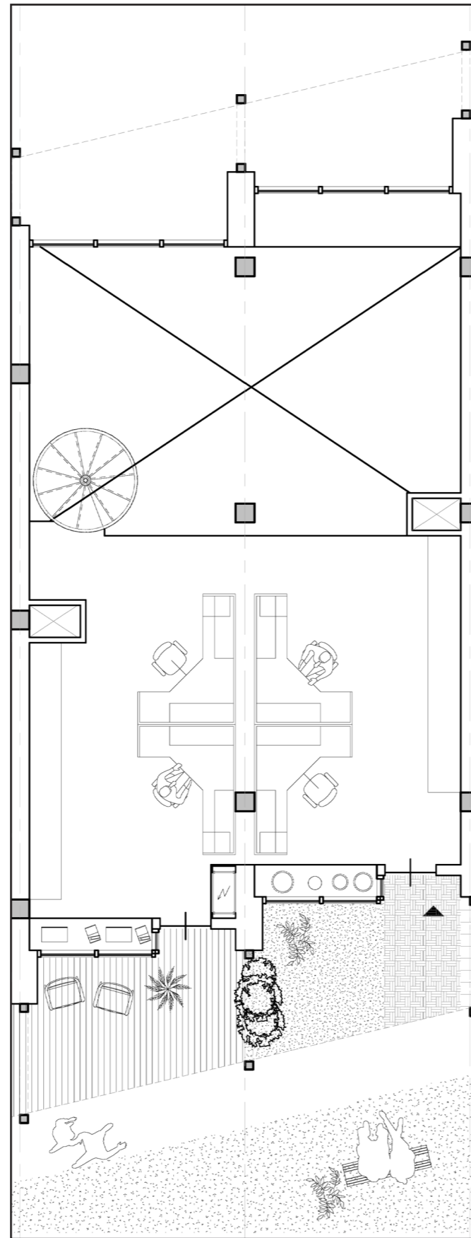
NouJIJ! - disassembly space 1:100
