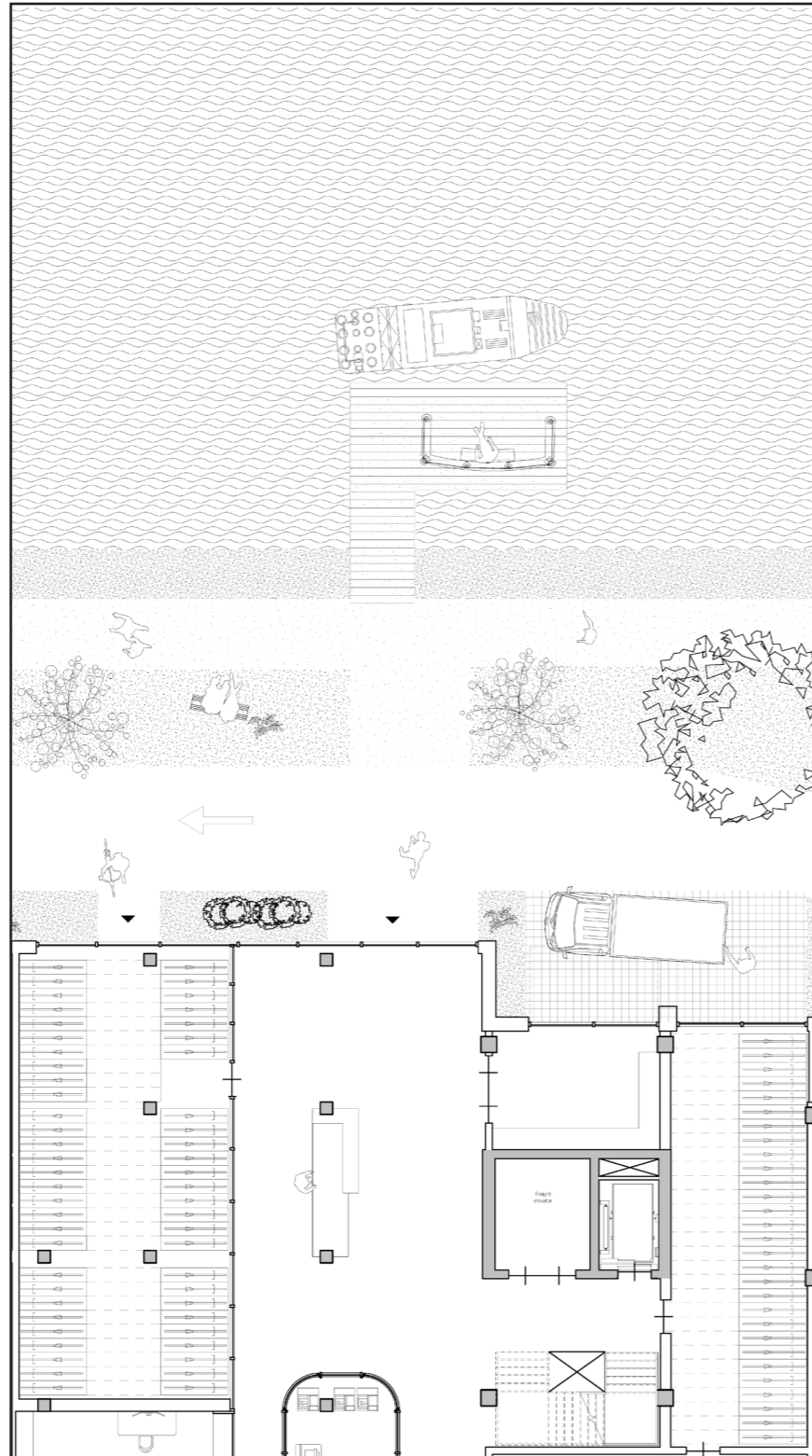
Boulevard 1:200
