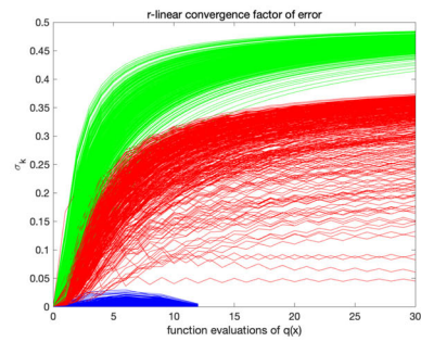
(d) Convergence factor
