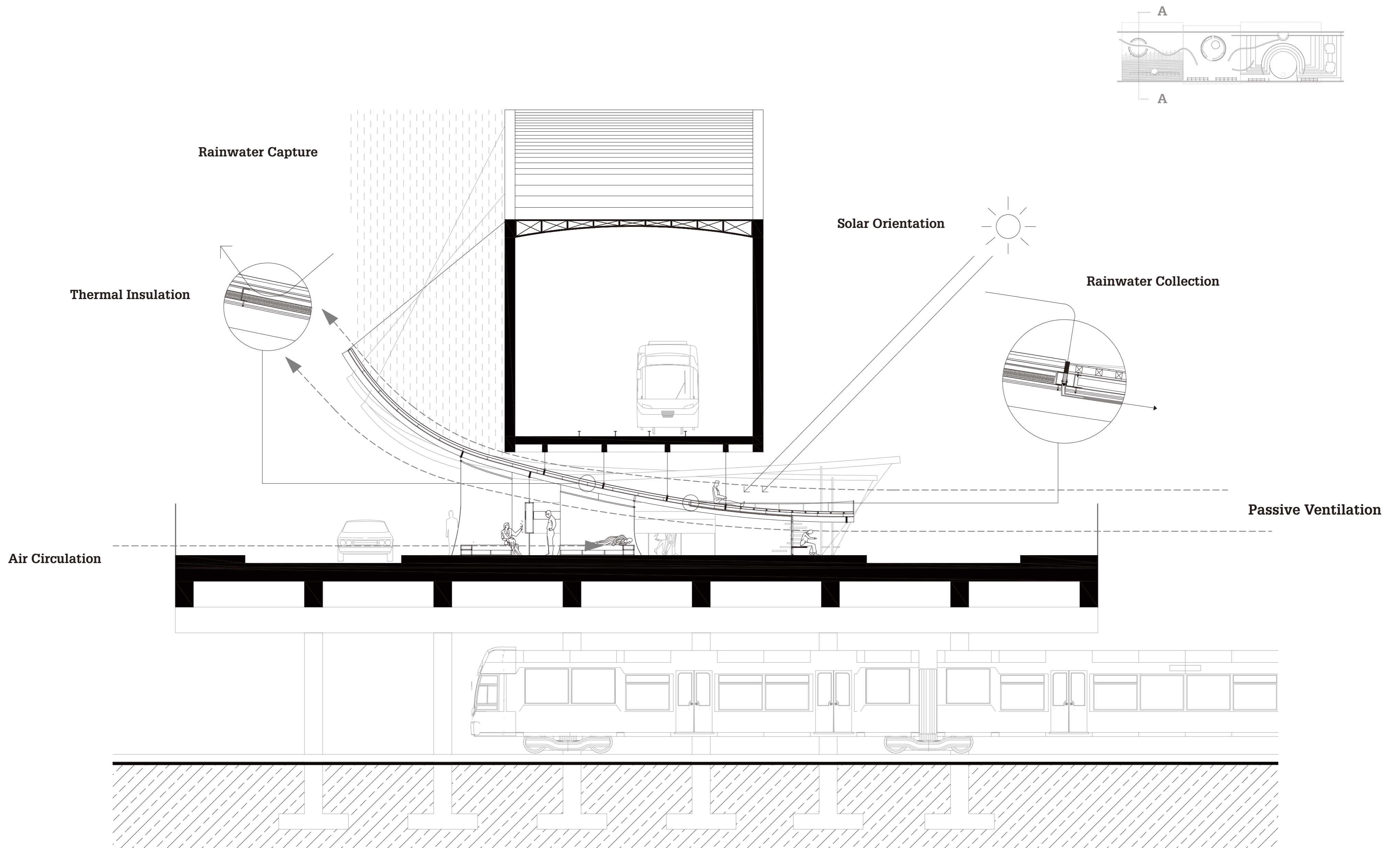
SECTION A-A 1:100
