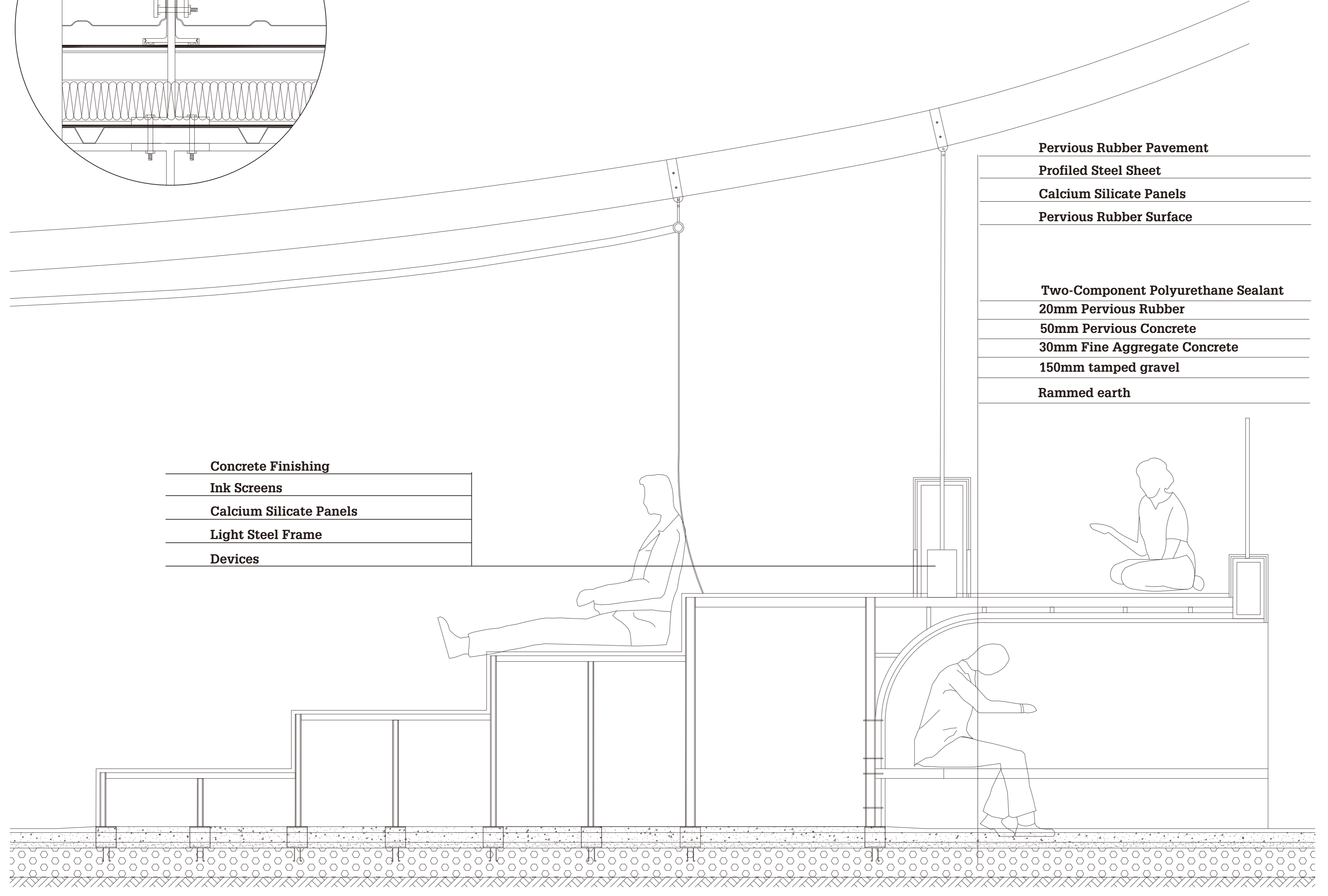
DETAIL C 1:15
